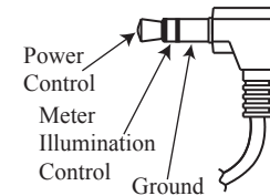
Figure 09– Power control (trigger) mini plug
